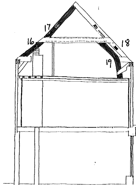
SECTION B-B TRUSS T.ii
