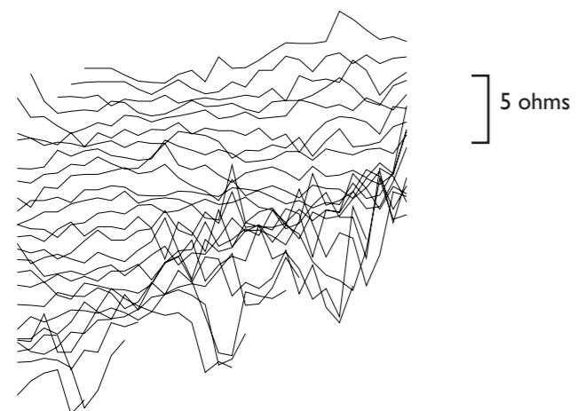
(D) Trace plot of minimally processed data
